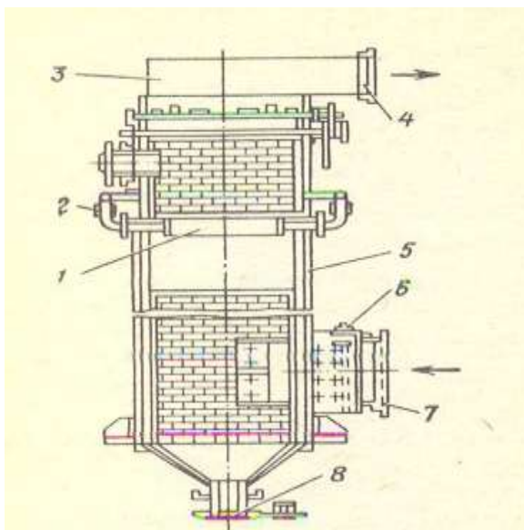
Surat Howany tozandan arassalaýjy enjamyň çyzgydy.
